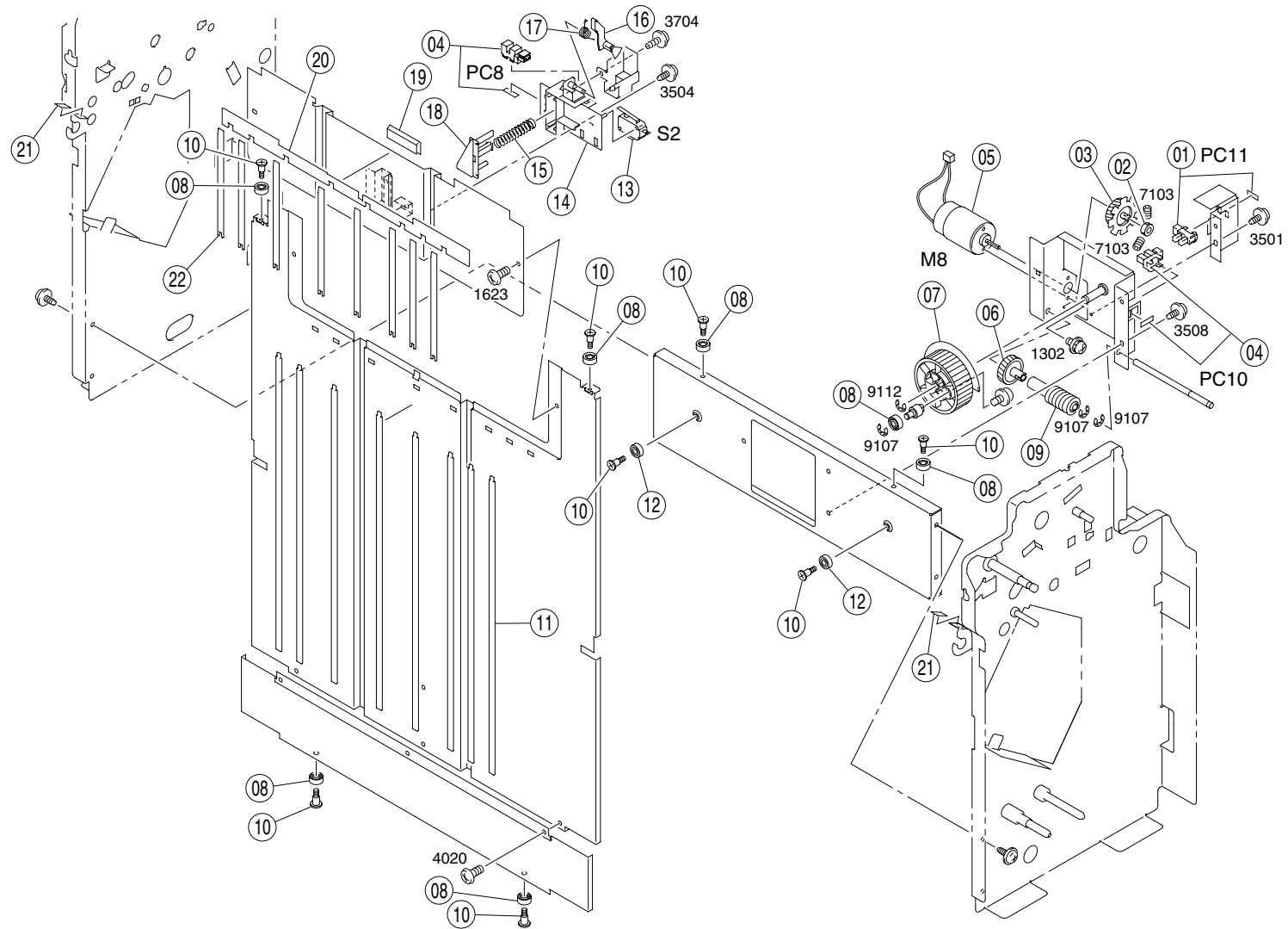
FIG. 10 SHIFT DRIVE
